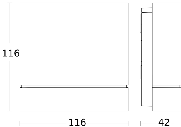
Maßzeichnung 1
